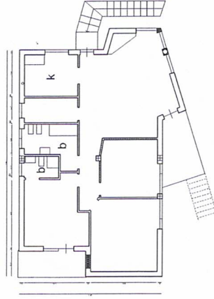
PIANTA ABITAZIONE
